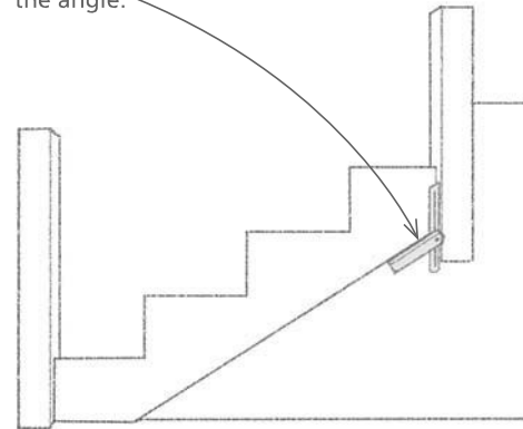
Skirtboard
